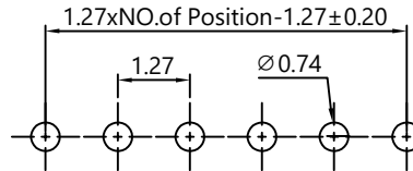
P.C.B Layout
