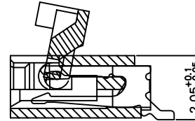
SECTION A-A (S=2:1)
