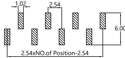
P.C.B Layout TYPE B
