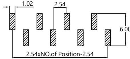
P.C.B Layout TYPE A
