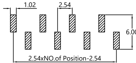
P.C.B Layout TYPE A
