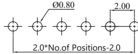
PCB LAOUT
