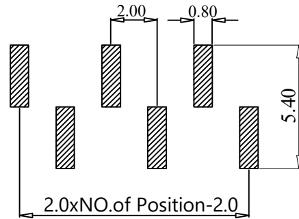
P.C.B Layout TYPE A
