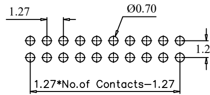
P.C.B Layout
