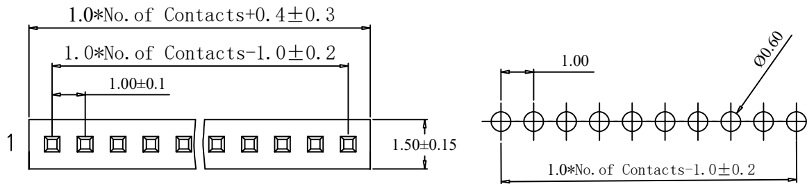
P.C.B Layout
