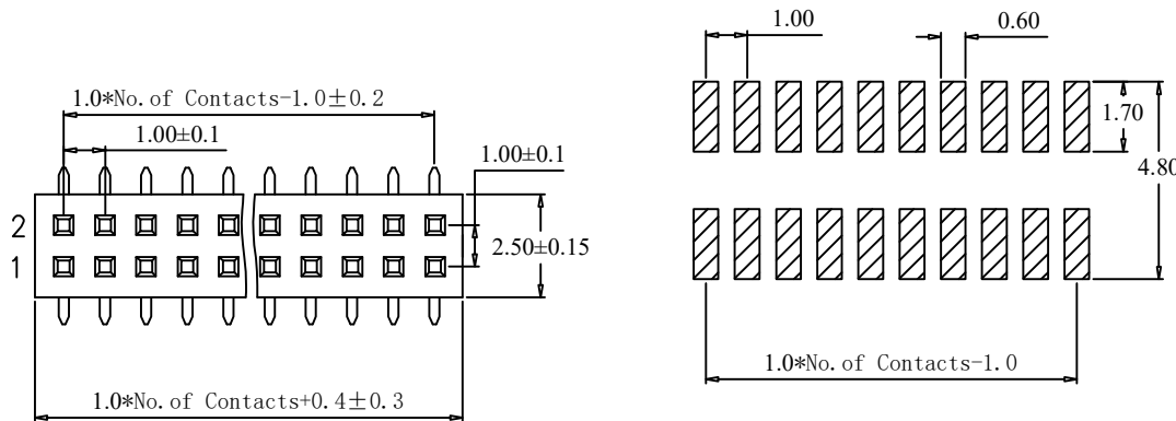
P.C.B Layout
